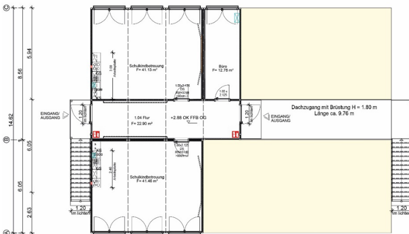
Obergeschoss
