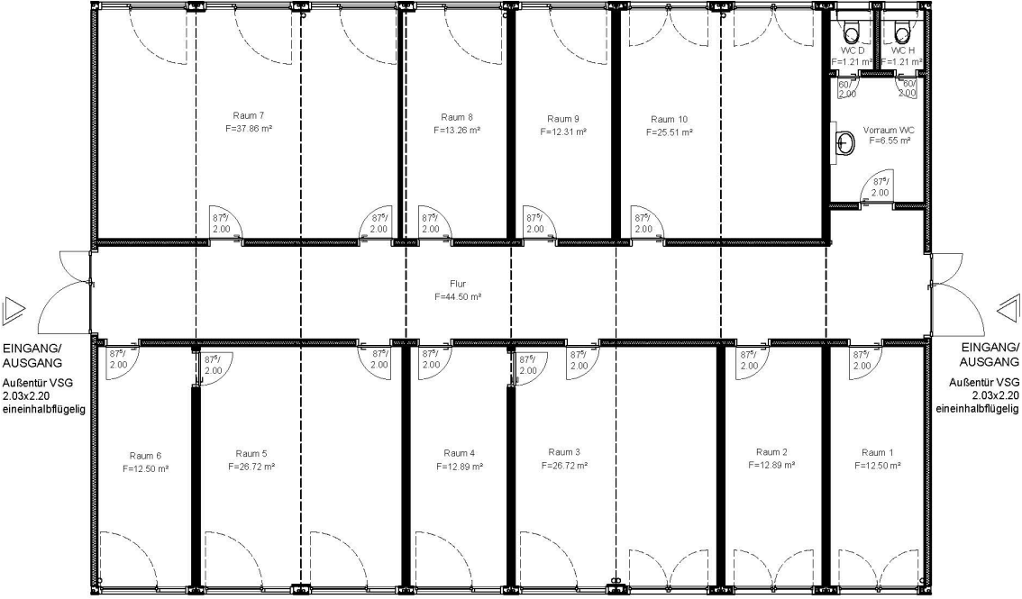
Erdgeschoss
